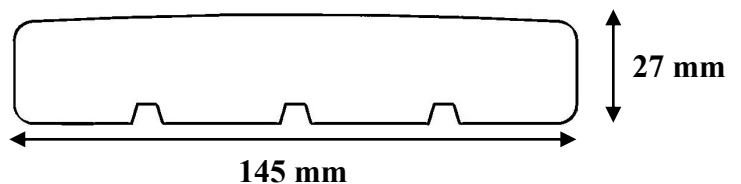
Lame profil bombé
